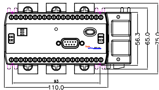
NEW-METER 치수
