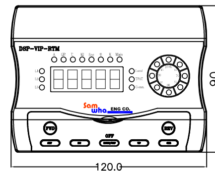
Old-METER 치수
