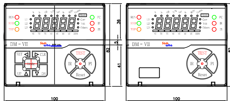
NEW-METER 치수
