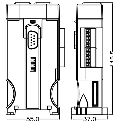
RS-485 통신모듈(레코드포함) 치수
