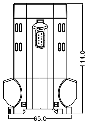
관통, 단자형 치수
