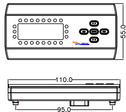
LOAD 치수
